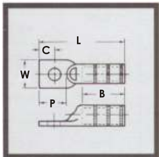
Zapatas de un barreno "Peep-Hole"
